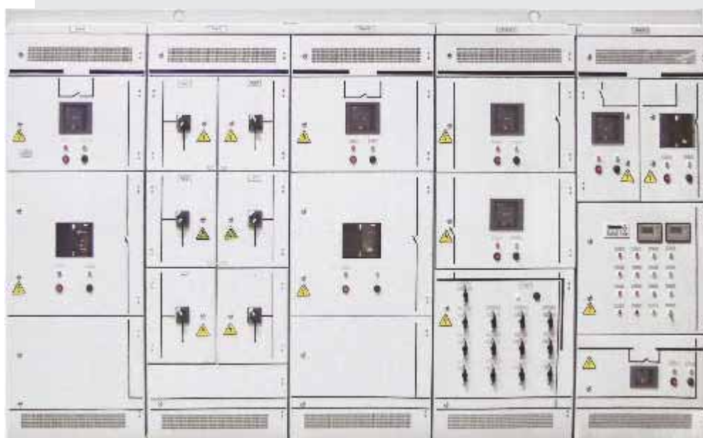
Фрагмент щита постоянного тока типа ШТЭ с микропроцессорным контроллером
