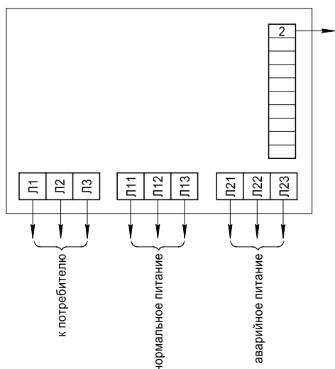
Схема подключения ящика управления ЯУ8351
