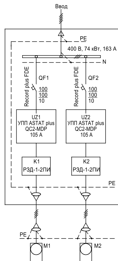
Шкаф УПП. Схема однолинейная.
