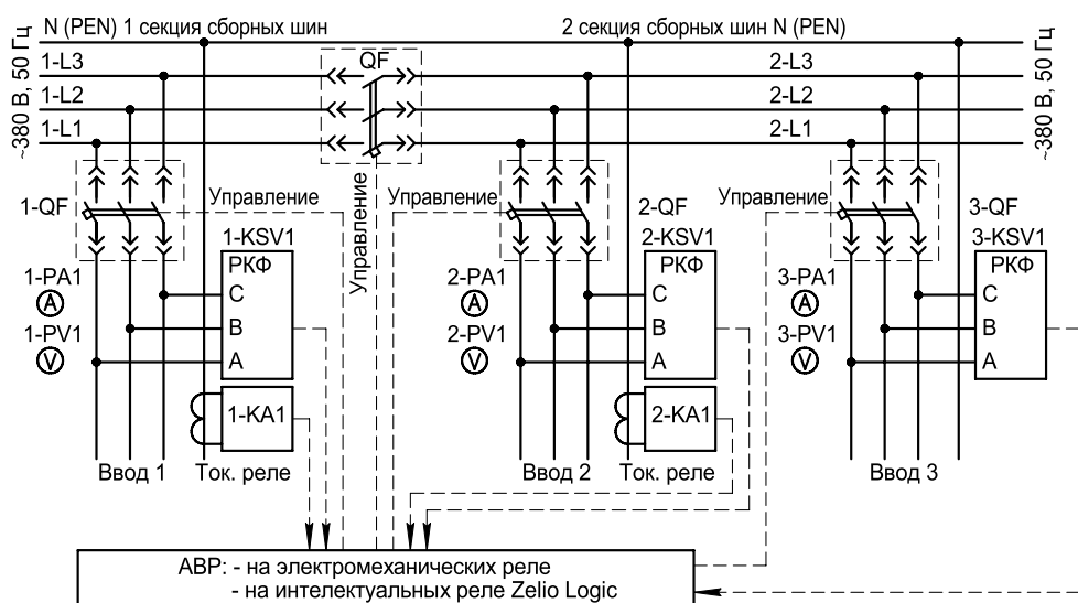
Структурная схема АВР на три ввода (3-ий ввод от ДЭС) с защитой от однофазного замыкания.
