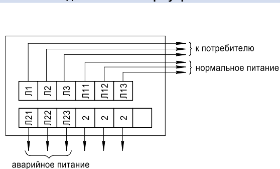
Схема подключения шкафа управления ШУ8253-32A2
