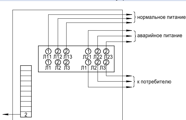
Схема подключения панели управления ПУ8253-52A2
