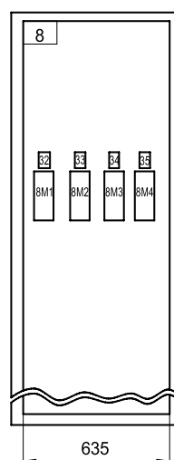
Дверь панели 4 Вид спереди
