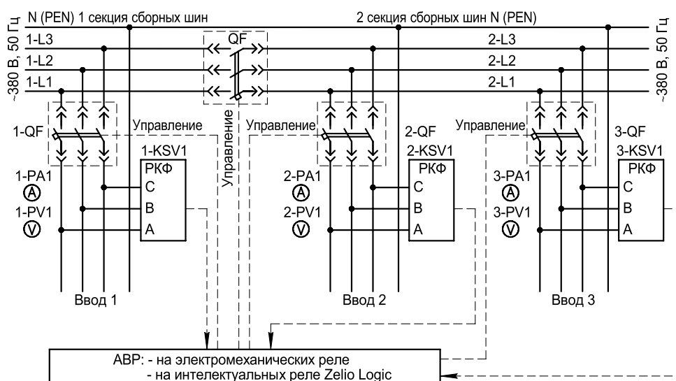
Структурная схема АВР на три ввода (3-ий ввод от ДЭС) без защиты от однофазного замыкания.
