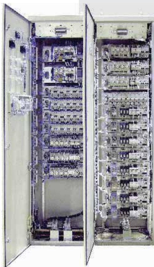
НКУ управления электроприводами задвижек серии РТЗО на базе оцинкованного конструктива
