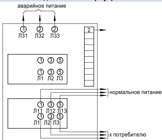
Схема подключения ящика управления ЯУ8254, ШУ8253-42A2 (52A2)
