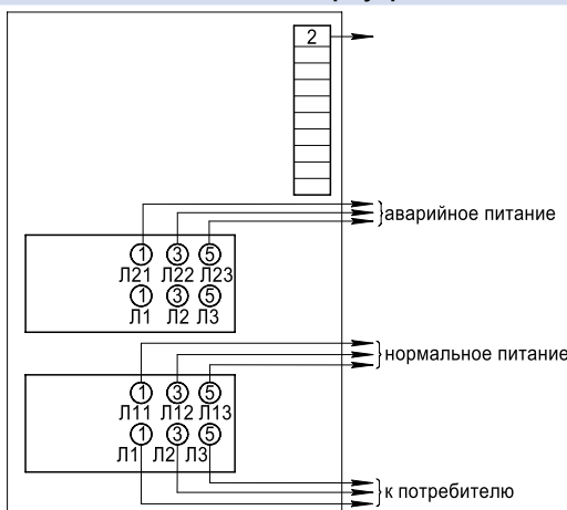
Схема подключения шкафа управления ШУ8254-62A2
