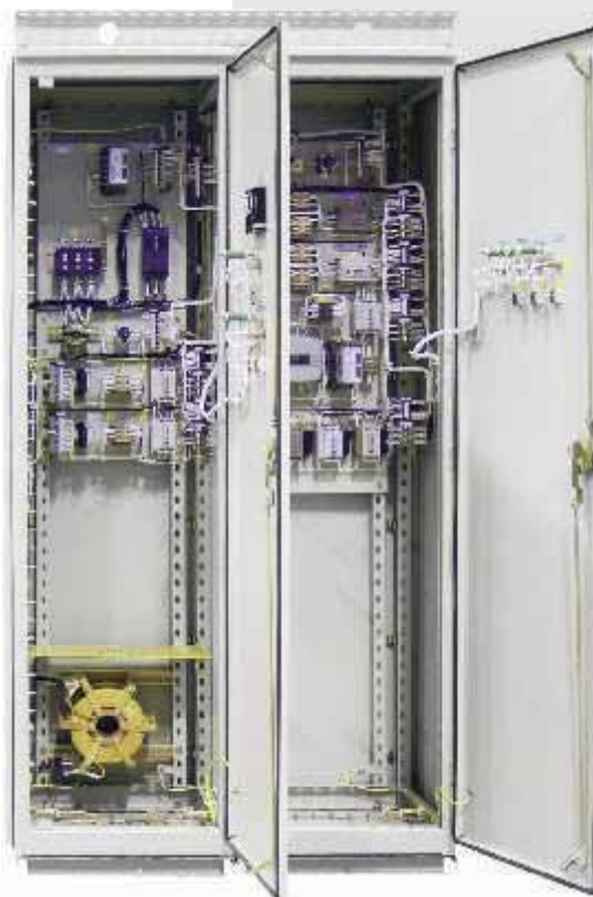
НКУ управления электроприводами системы топливоподдачи УРСН-50М, УРСН-600М
