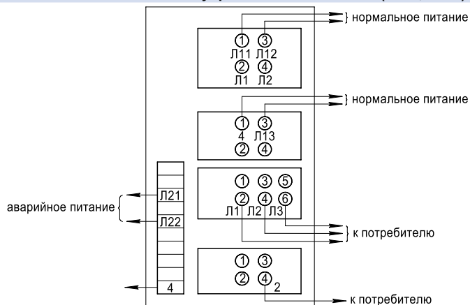
Схема подключения шкафа управления ШУ8253-32A2
