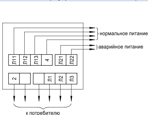
Схема подключения шкафа управления ШУ8255-22A2 (32A2, 42A2)
