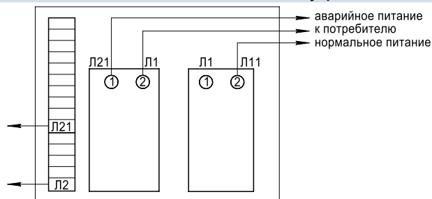
Схема подключения панели управления ПУ8253-52A2
