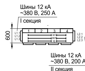
Вид сверху М1:50
