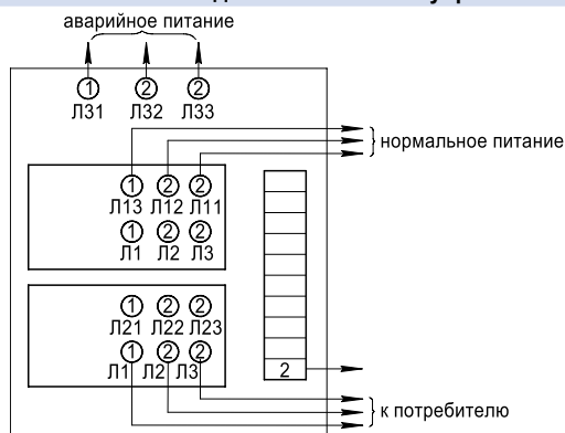
Схема подключения шкафа управления ШУ8254-62A2
