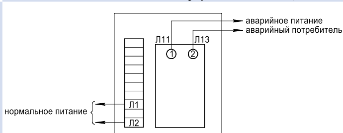
Схема подключения панели управления ПУ8255-22A2(32A2, 42A2)
